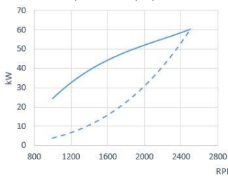
Puissance (ISO 3046/1)
